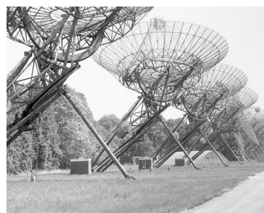
荷兰射电天文研究所
